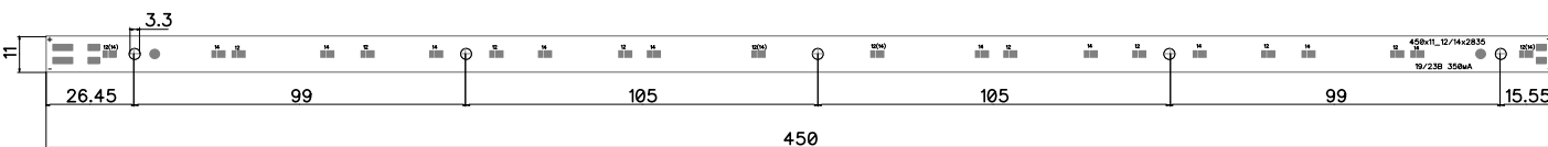
Габаритный чертеж модуля 16-22 диодов
