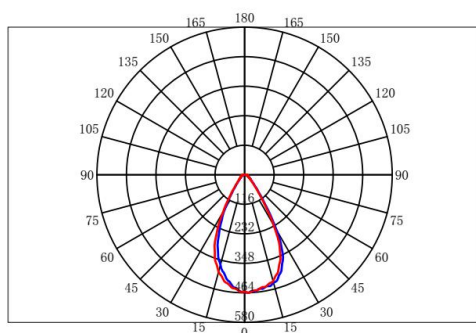
配光曲线
