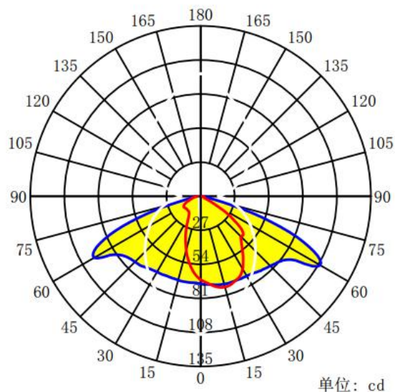
配光曲线
