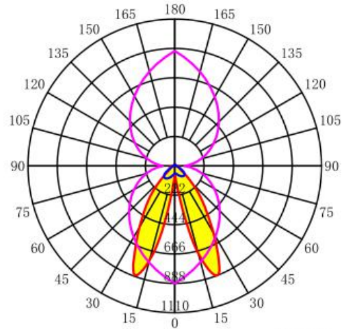
配光曲线
