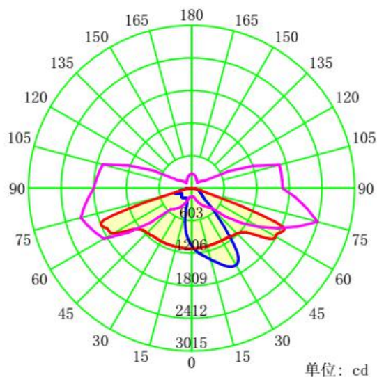
配光曲线
